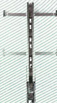
Bild 6: Führung mit Kupplungsstück, Typ: MH-AL (Aluminium)
